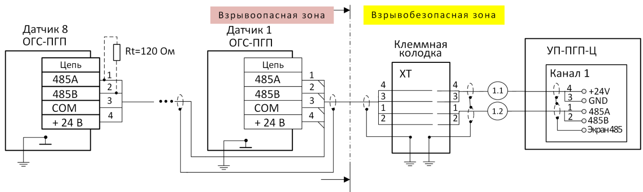
Одноименные контакты разъемов X2 и X3 соединены на клеммной плате Рисунок А.3 – Схема электрическая подключения газоанализатора по RS-485
