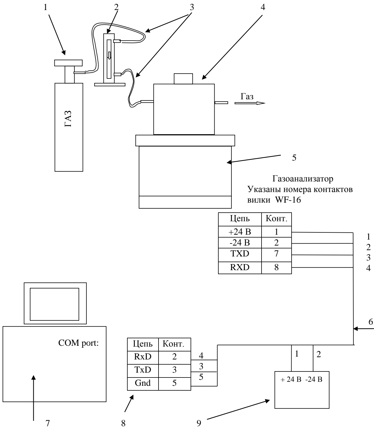
Рисунок Б.1 - Схема соединений для установки «нуля» и калибровки газоанализатора при помощи компьютера.
